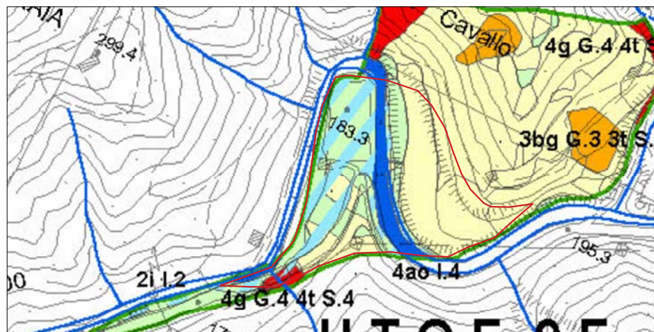
Figura 8 - Carta Pericolosità Geologica, Idraulica e Sismica R.U. 2010 1:5.000
